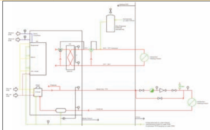
Schnittstellen und Abrechnung Heizwassersystem, Dampfsystem, Kondensat und Wasser
